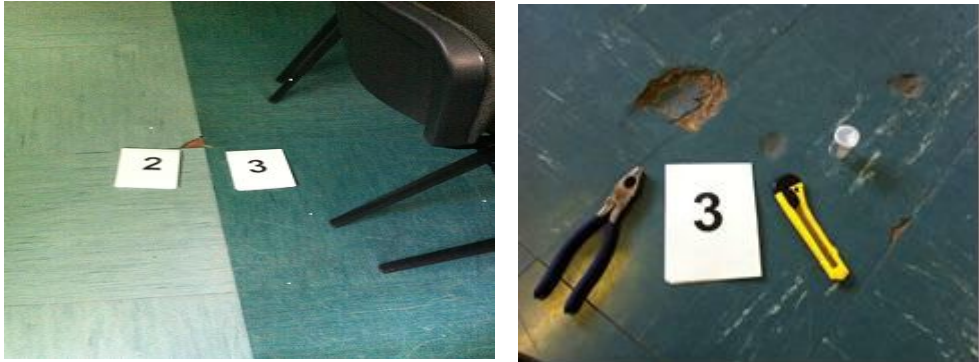
Figure 39 - esempio di prelievo campione pavimentazione in vinil-amianto
