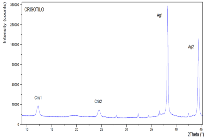
Figura 58 - diffrattogramma del crisotilo deposto su filtro d'argento
