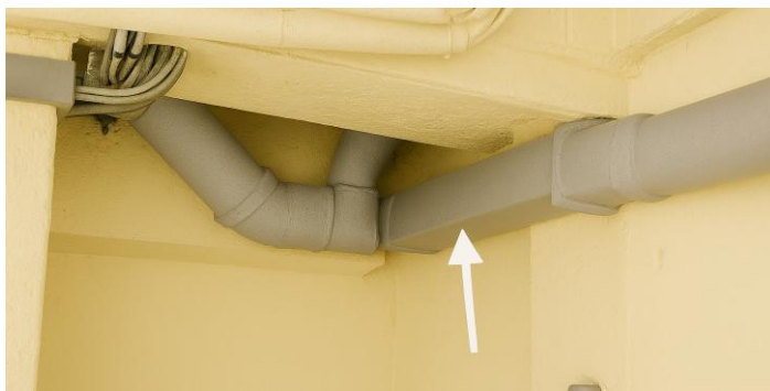
Figura 10 - canali di ventilazione in cemento-amiante
