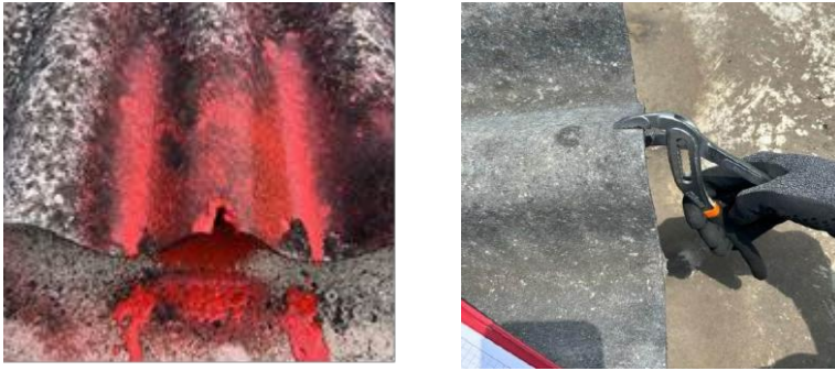
Figure 41 - prelievo del campione (dx) e sigillatura dell'area interessata (sx)
