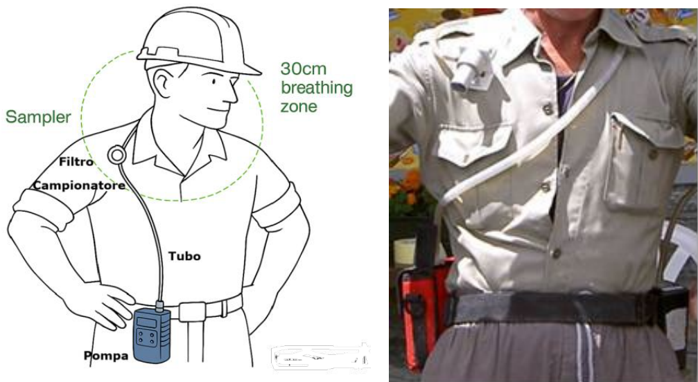
Figura 51 - campionamento personale con schema
