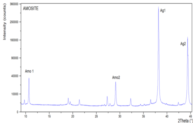
Figura 59 - diffrattogramma dell'amosite deposto su filtro d'argento
